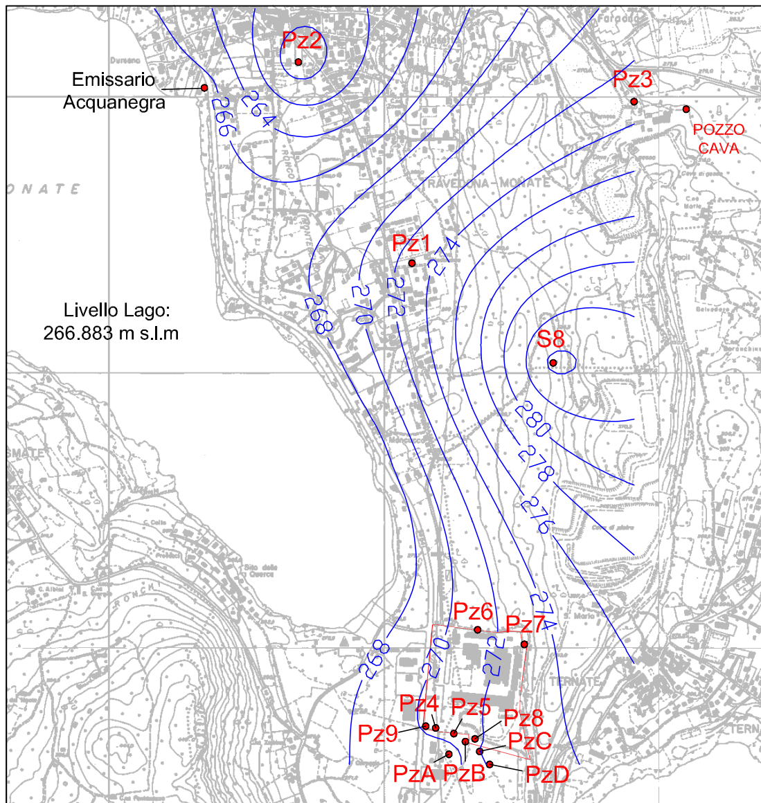
Figura 3: andamento piezometrico marzo 2014
