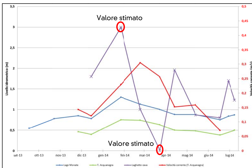
Grafico 11: correlazioni battenti idrici/velocità deflusso
