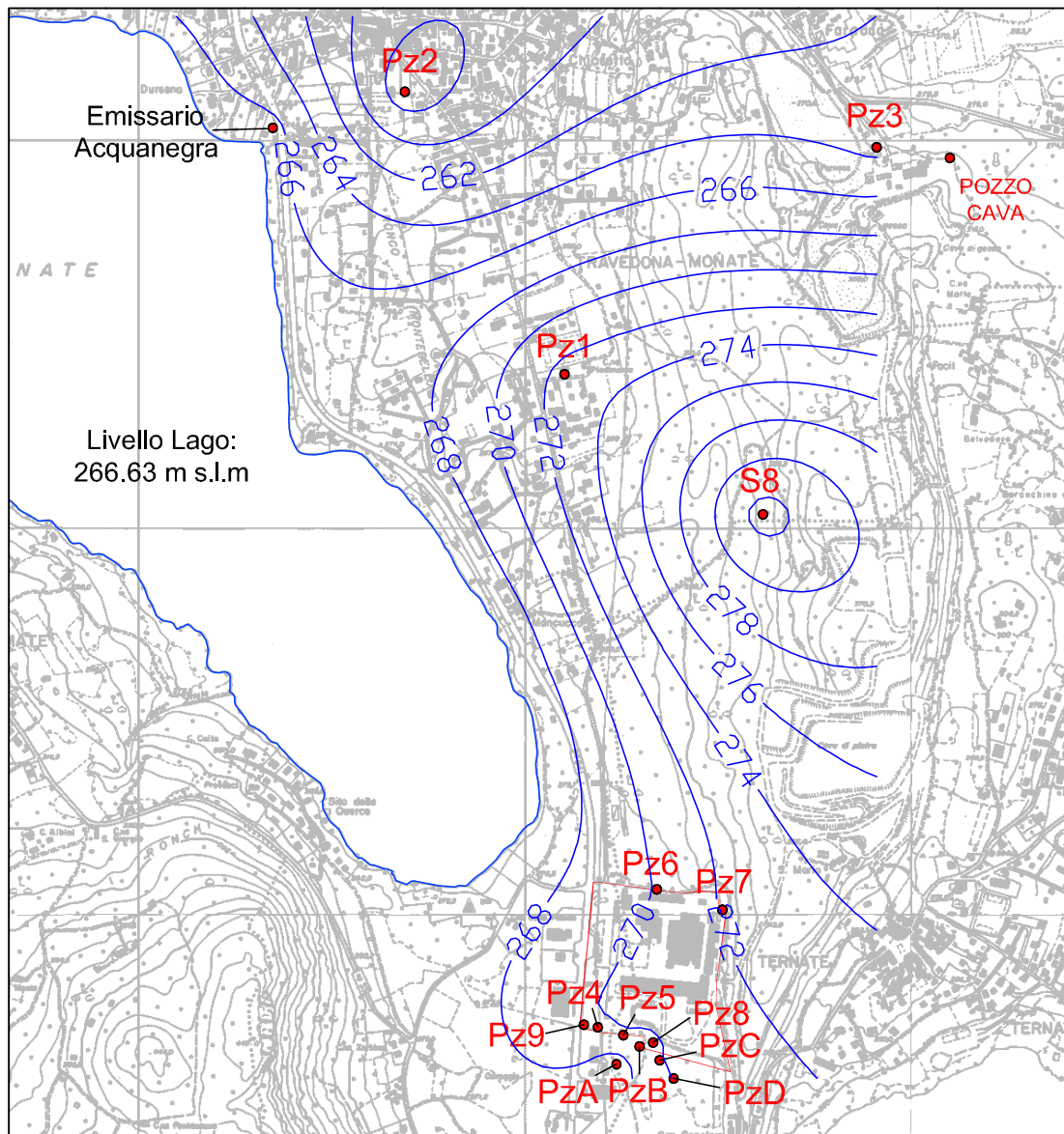
Figura 6: andamento piezometrico giugno 2014
