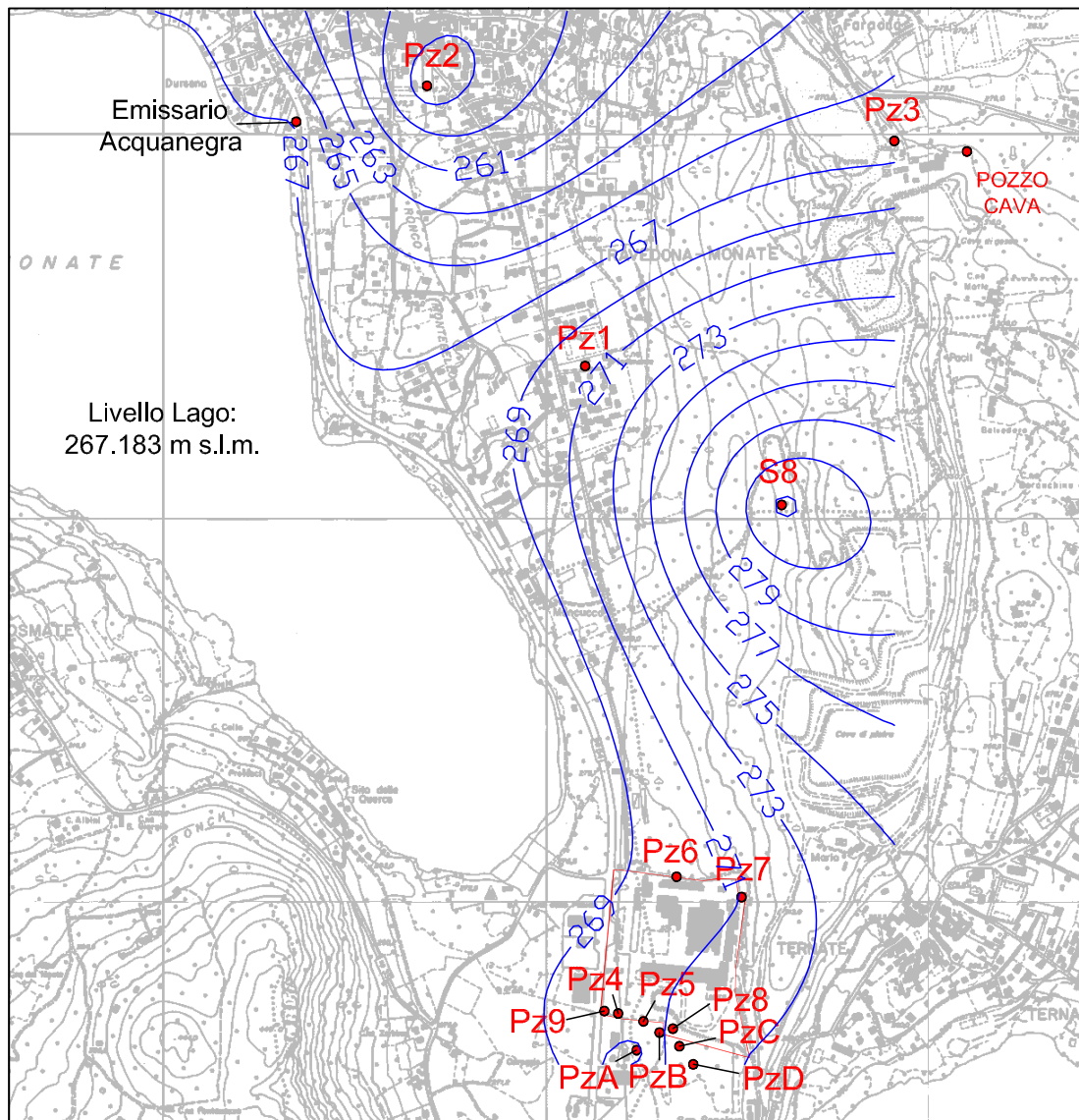
Figura 1: andamento piezometrico gennaio 2014
