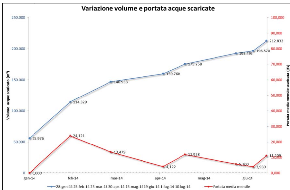
Grafico 13: portate emunte dal laghetto di cava
