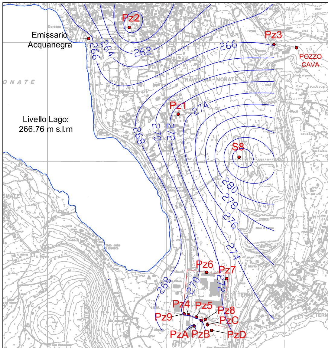
Figura 5: andamento piezometrico maggio 2014
