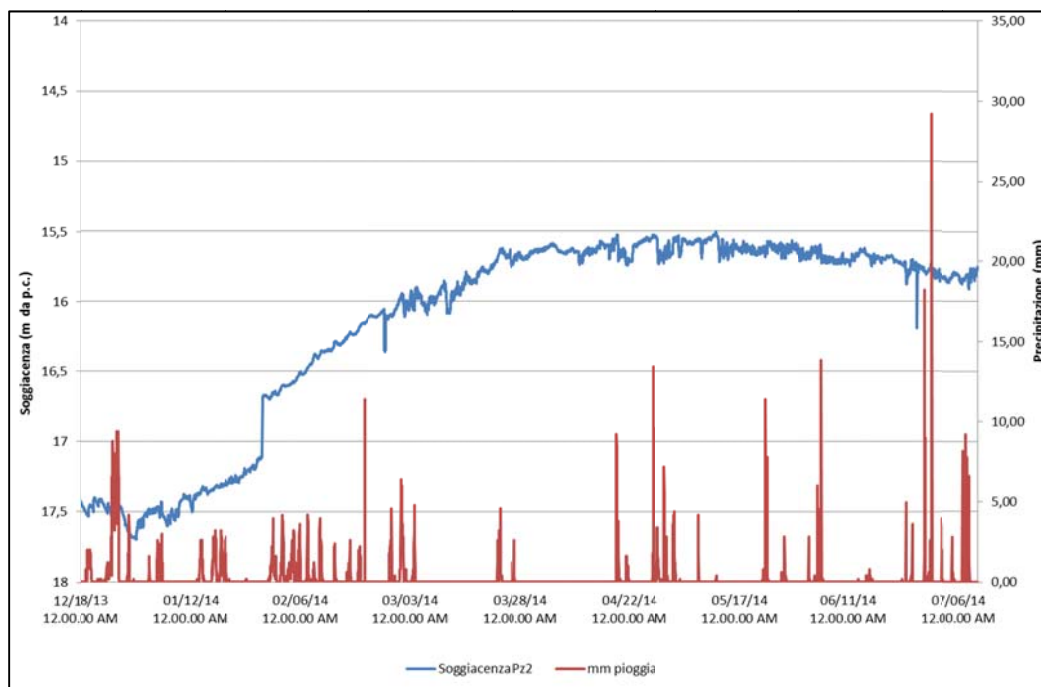
Grafico 4: Correlazione tra dati pluviometrici e soggiacenza - Pz2
