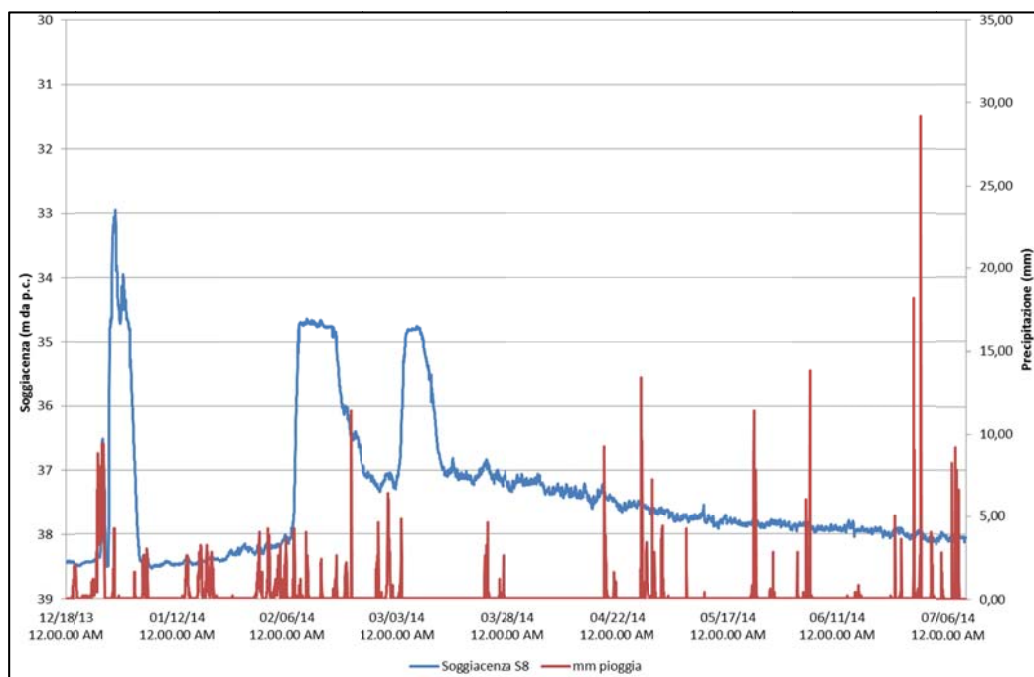
Grafico 8: Correlazione tra dati pluviometrici e soggiacenza - S8
