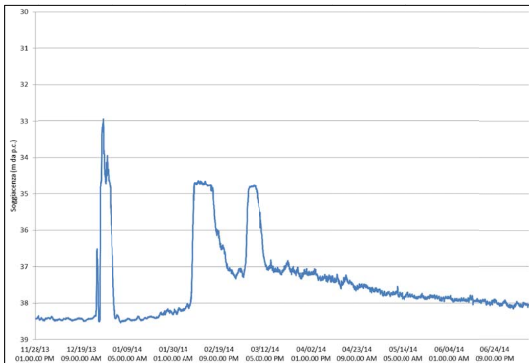
Grafico 7: oscillazione della superficie piezometrica registrata nel piezometro S8 (novembre 2013 – luglio 2014)
