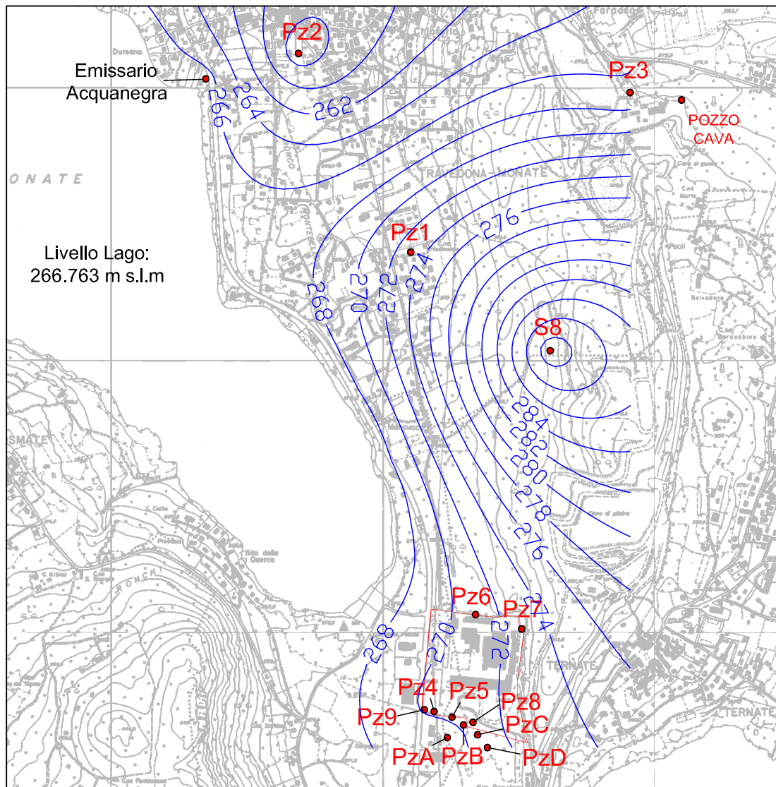
Figura 4: andamento piezometrico aprile 2014
