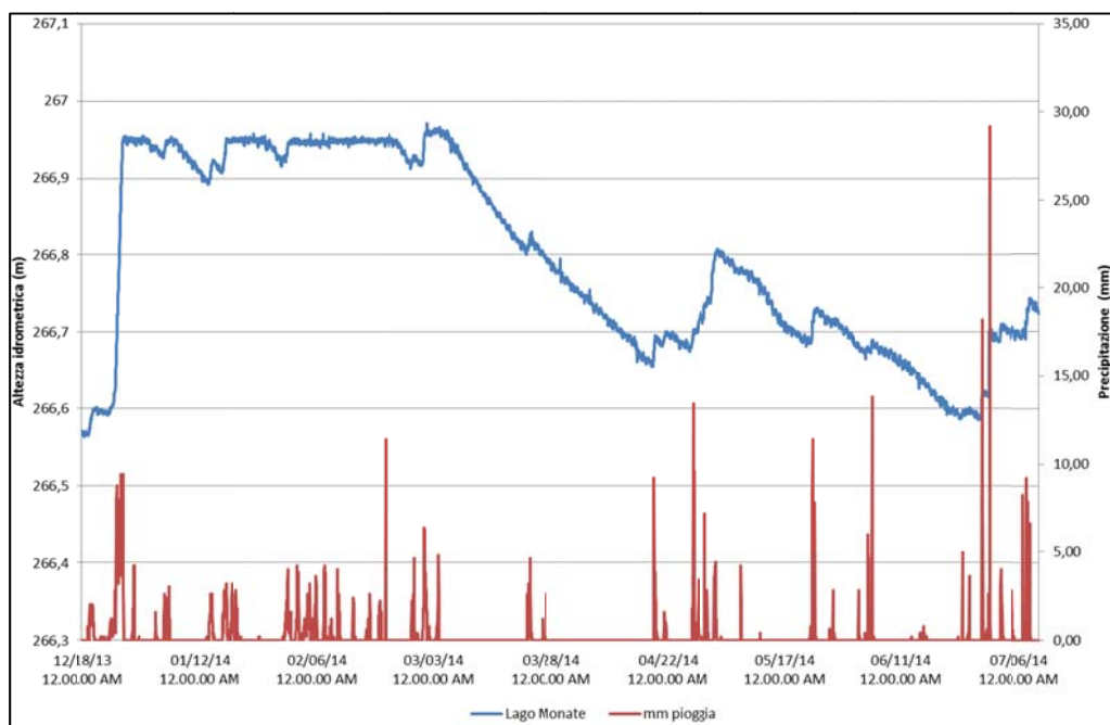
Grafico 10: Correlazione tra dati pluviometrici e andamento idrometrico Lago di Monate
