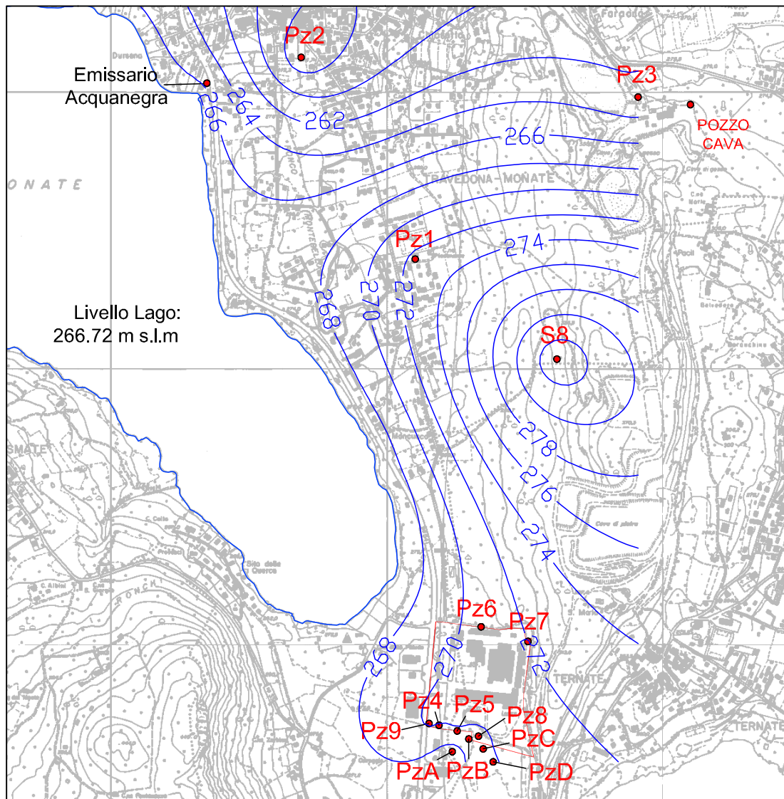
Figura 7: andamento piezometrico 1 luglio 2014
